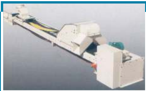
Förderband mit Abwurfwagen
